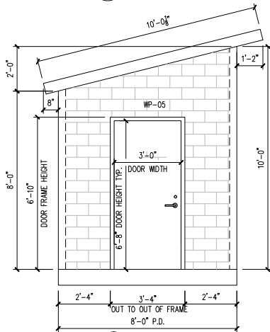
(D) LEFT ELEVATION
